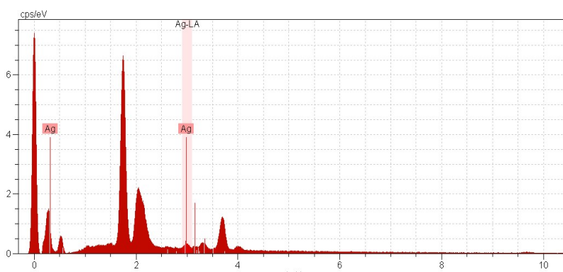
نمودار ۳ و شکل ۲- نمودار و MAP پراکنندگی نقره بر اساس لایه L الکترونی اتم نقره برای نمونه SBMP-H
