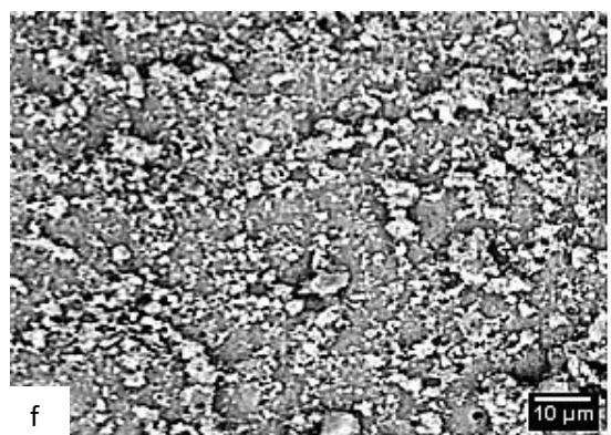
شکل ۱- نمونه تصاویر میکروسکوپ الکترونی گروه‌های مختلف با بزرگنمایی \times 4500 -a- خمیردندان فلورایددار ۳ روزه، -b- خمیردندان فلورایددار ۷ روزه، -c- خمیردندان فلورایددار ۱۴ روزه، -d- ۳ روزه CHA خمیردندان، -e- ۷ روزه CHA خمیردندان، -d- ۱۴ روزه CHA خمیردندان
