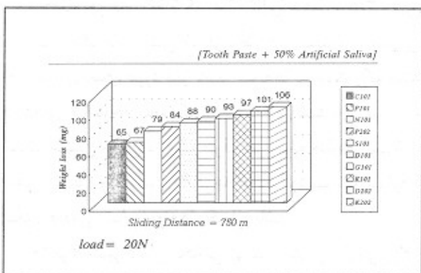
تصویر شماره ۶- مقایسه مقدار سایش آمالگام تولید داخلی A_2 در یک مسافت خاص طی اجرای آزمونهای سایش سه جسمی با چند نوع خمیر دندان
