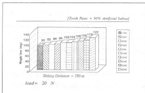
تصویر شماره ۸- مقایسه مقدار سایش آمالگام تولید خارجی A 4 در یک مسافت خاص طی اجرای آزمونهای سایش سه جسمی با چند نوع خمیر دندان
