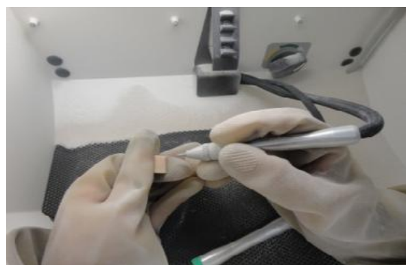
شکل ۲- عمل سندبلاست
