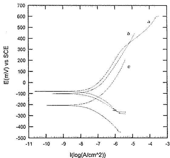
تصویر ۷- نمودارهای پلاریزاسیون کاتدی و آندی سه نوع زیرلایه فلزی با پوشش هیدروکسی آپاتیت a- فولاد زنگ‌نزن ۲۱۶ ال با پوشش b- آلیاز وایتالیوم با پوشش c- تیتانیوم خالص تجارتي با پوشش، در محلول رینگر در دمای ۳۷ درجه سانتیگراد
