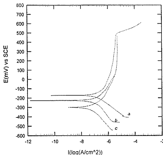
تصویر ۶- نمودارهای پلاریزاسیون کاتدی و آندی سه نوع زیرلایه فلزی بدون پوشش a- فولاد زنگ‌نزن ۲۱۶ ال b) آلیاز وایتالیوم c- تیتانیوم خالص تجارتي، در محلول رینگر در دمای ۳۷ درجه سانتیگراد
