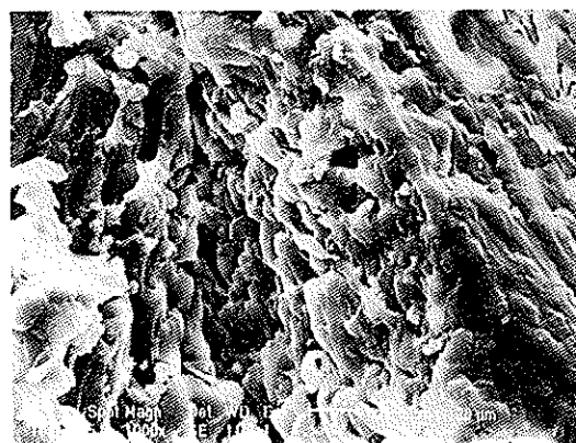
تصویر ۳- نمایی از مخلوط رزین آکریلی با ذرات Al_2O_3 (بزرگنمایی ۱۰۰۰ برابر)
