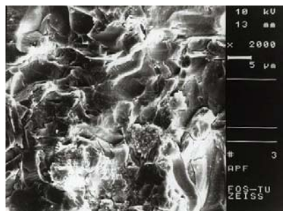
شکل ۵- فتومیکروگراف سطح پرسن اچ شده با APF ۲۳٪ به مدت ۱۰ دقیقه (بزرگنمایی ۲۰۰۰ برابر)
