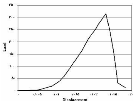
شکل ۱- منحنی رفتاری (نیرو- تغییر شکل) نمونه‌ای از گروه اول در آزمون DTS
