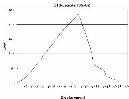
شکل ۲- منحنی رفتاری (نیرو- تغییر شکل) نمونه‌ای از گروه دوم در آزمون DTS
