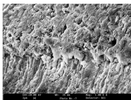
شکل ۵- گروه پنجم شستن آلودگی با NaOCl و استفاده مجدد از ادهزیو؛ وجود interlocking در فصل مشترک ماده ترمیمی و عاج مشهود است.
