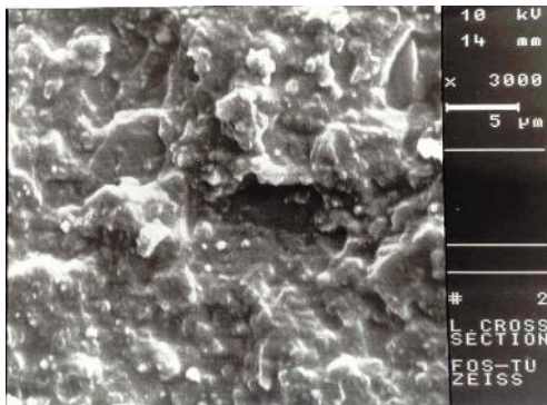
شکل ۲- نمای SEM از سطح شکست کامپوزیت لوسیت
