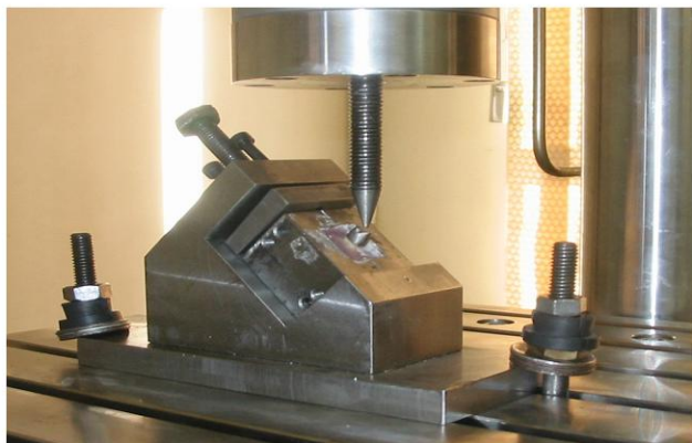
شکل ۳- نمونه‌ها در زیر دستگاه Zwick میلی‌متری
