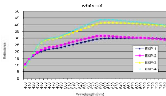
شکل ۲- نمودار انعکاس نور گروه‌ها به عنوان یک تابعی از طول موج در زمینه سفید
