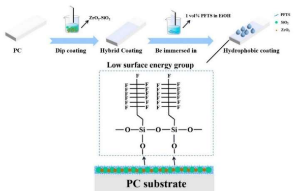
شکل ۲- شماتیک پوشش سل‌ژل هیبریدی زیرکونیا/سیلیکا همراه با لایه نهایی با انرژی سطحی پایین (۱۱)
