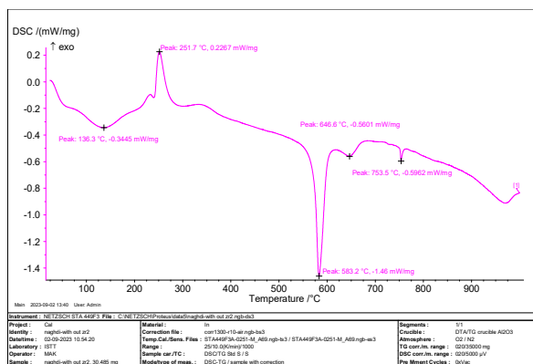
نمودار ۱- نمودار آزمون حرارتی کالریمتری تفاضلی روبشی
