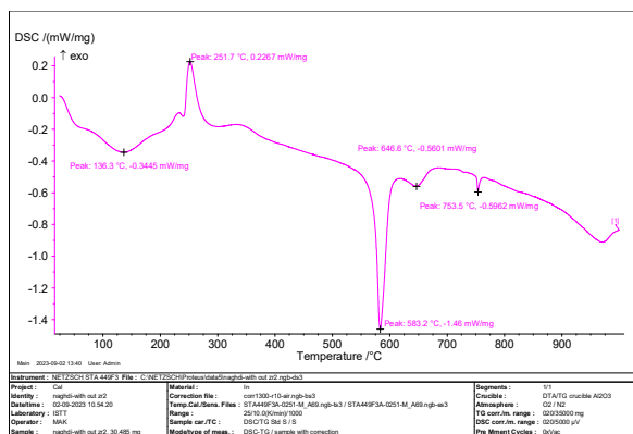
نمودار ۱- نمودار آزمون حرارتی کالریمتری تفاضلی روبشی
