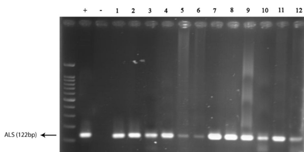
شکل ۱- ژل الکتروفورز محصول آزمون PCR از چپ به راست: Ladder 100bp- کنترل مثبت (کاندیدا آلیکنس حاوی ژن مورد نظر)- کنترل منفی (آب مقطر)- آغازگر اختصاصی ALS (122 bp)
