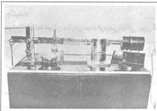
تصویر شماره ۱- دستگاه اندازه‌گیری سایش با روش میله بر روی صفحه
