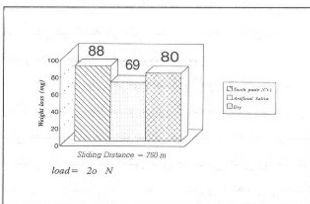
تصویر شماره ۳- نمودار مقایسه مقدار سایش آمالگام تولید داخلی A_1 در سه حالت خشک، همراه با خمیر دندان و همراه بزاق مصنوعی در تماس با چینی طی آزمون به روش میله بر روی صفحه
