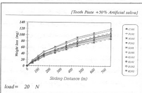
تصویر شماره ۴- نمودار کاهش وزن (مقدار سایش) آمالگام تولید داخلی A_1 بر حسب مسافت طی شده (طول فاصله تماس) در آزمون سایش سه جسمی با استفاده از خمیر دندان
