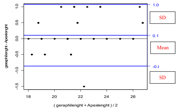
شکل ۲- نمودار Bland-Altman برای بررسی توافق میان مقادیر اندازه‌گیری شده، میزان طول کانال ریشه به وسیله اپکس یاب و پرتونگاری در همه دندان‌ها
