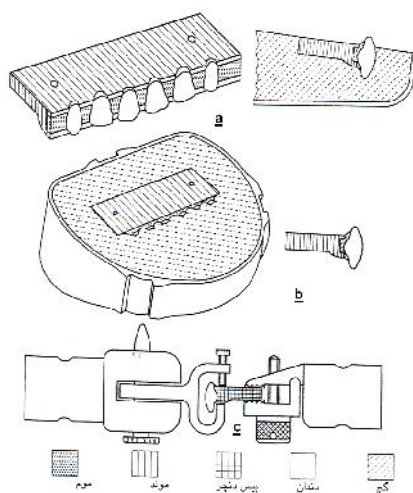
شکل ۴- قالب فلزی
