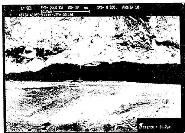
تصویر شماره ۳- سطح باکال در نمونه با کلار با بزرگنمایی ۵۰۰ برابر در مرحله بعد از گلیز
