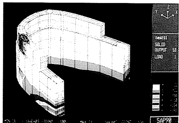
تصویر شماره ۱- توزیع تنش در قوس مربعی نرمال به هنگام اعمال نیروی یک‌طرفه عمودی
