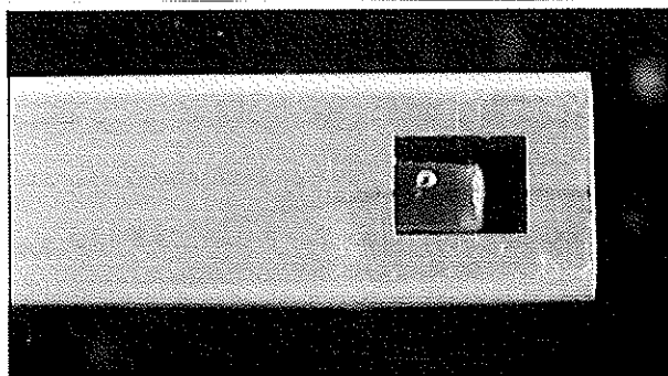
تصویر ۵- آزمایش انبساط حرارتی در دمای 40^\circ\text{C} ساتیگراد (اولیه)
