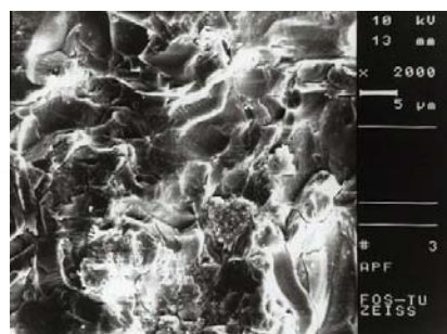
شکل ۵- فتومیکروگراف سطح پرسلن اچ شده با APF ۱/۲۳٪ به مدت ۱۰ دقیقه (بزرگنمایی ۲۰۰۰ برابر)
