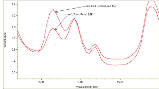
شکل ۳- طیف ScotchBond MP قبل و بعد از پلیمریزه شدن
