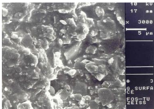
شکل ۴- نمای SEM از سطح شکست کامپوزیت شیشه
