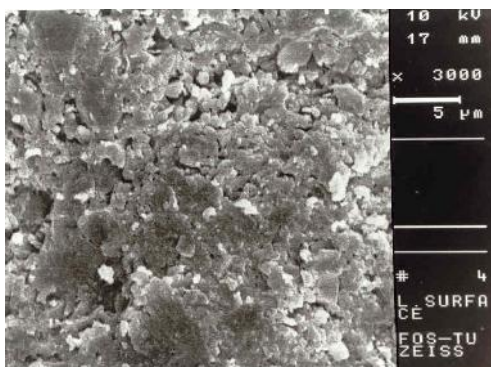
شکل ۳- نمای SEM از سطح سایش کامپوزیت لوسیت
