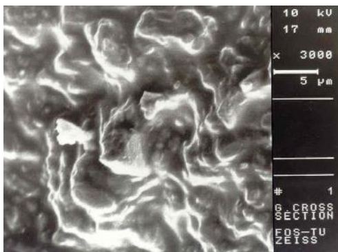
شکل ۴- نمای SEM از سطح شکست کامپوزیت شیشه
