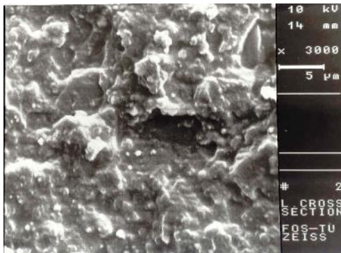
شکل ۲- نمای SEM از سطح شکست کامپوزیت لوسیت
