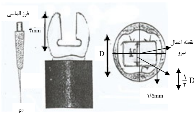
شکل ۱- طرح شماتیک تراش حفره
