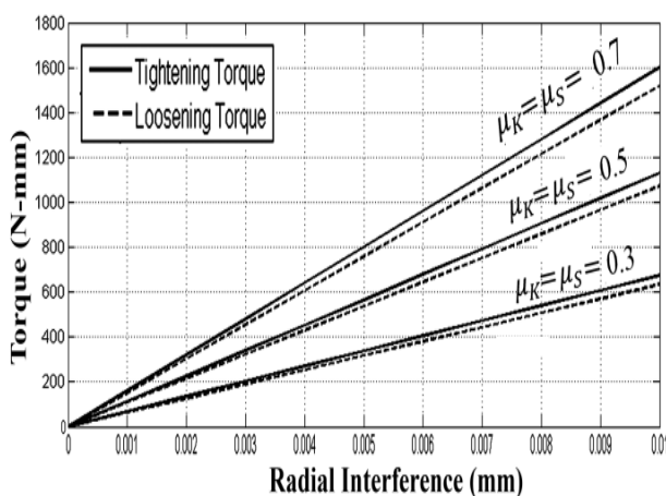
شکل ۴- تداخل شعاعی بر حسب گشتاور
